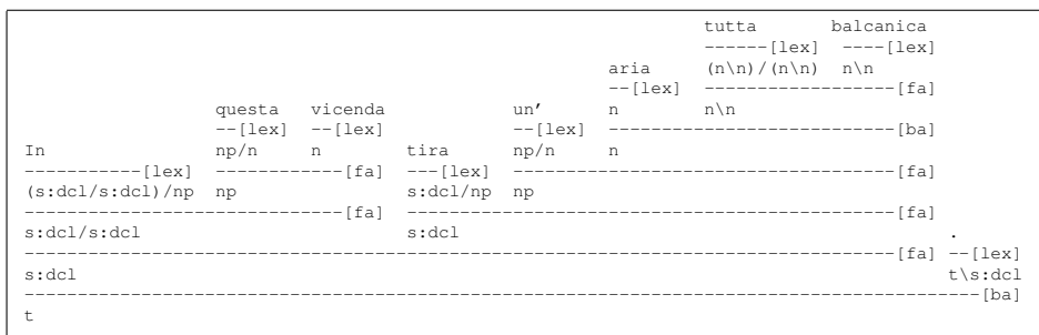
Figure 1: CCG derivation for In questa vicenda tira un' aria tutta balcanica .
