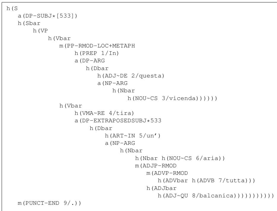
Figure 3: ConsTUT tree for In questa vicenda tira un' aria tutta balcanica .
